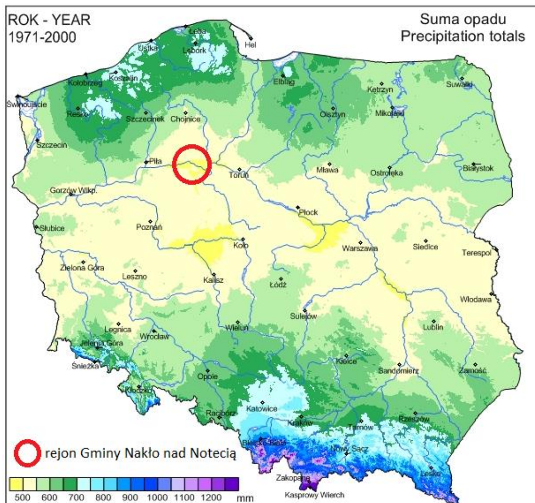
Ryc. 11. Roczne sumy opadów deszczu w latach 1971 - 2000
